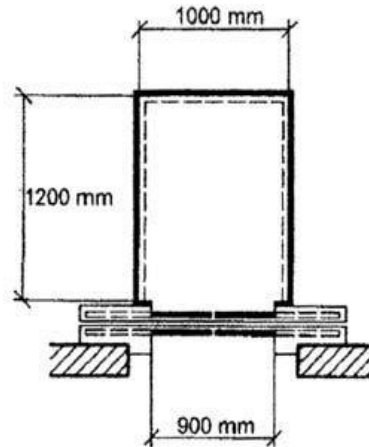
FIGURA 2. Dimensiones
