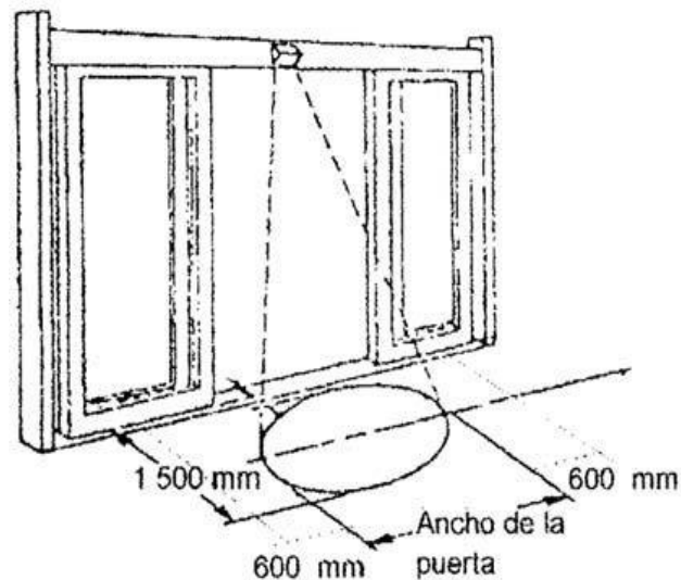
FIGURA 2. Puerta automática
