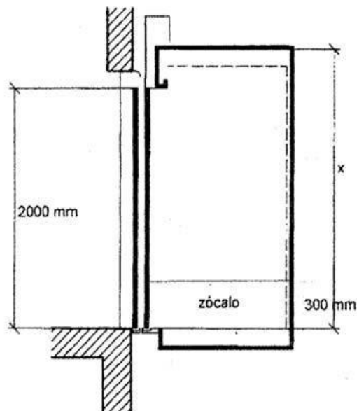
FIGURA 2. Dimensiones
