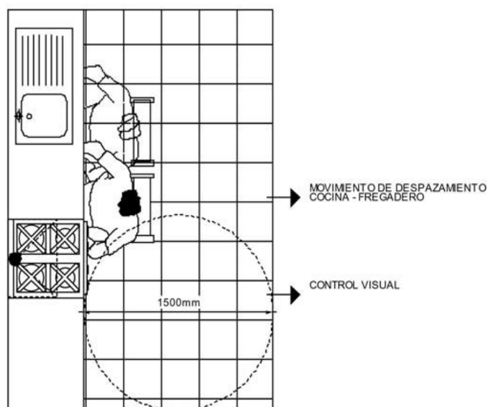
FIGURA 1.- ESPACIO LIBRE DE MANIOBRA DE GIRO
