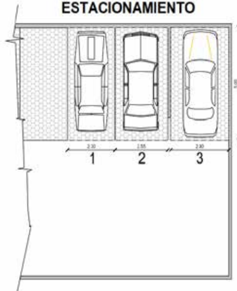
GRÁFICO 6: ANCHOS MÍNIMOS DE ESTACIONAMIENTO
