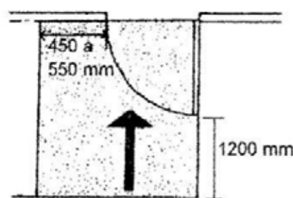
FIGURA 5. Espacios de acceso
