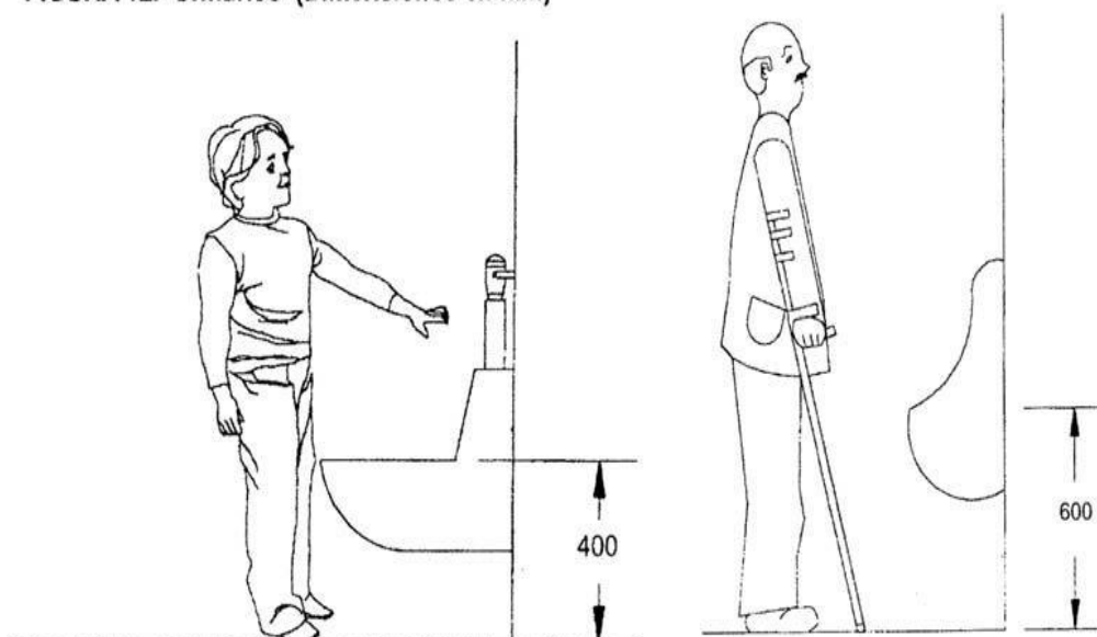
FIGURA 12. Urinarios (Dimensiones en mm)
