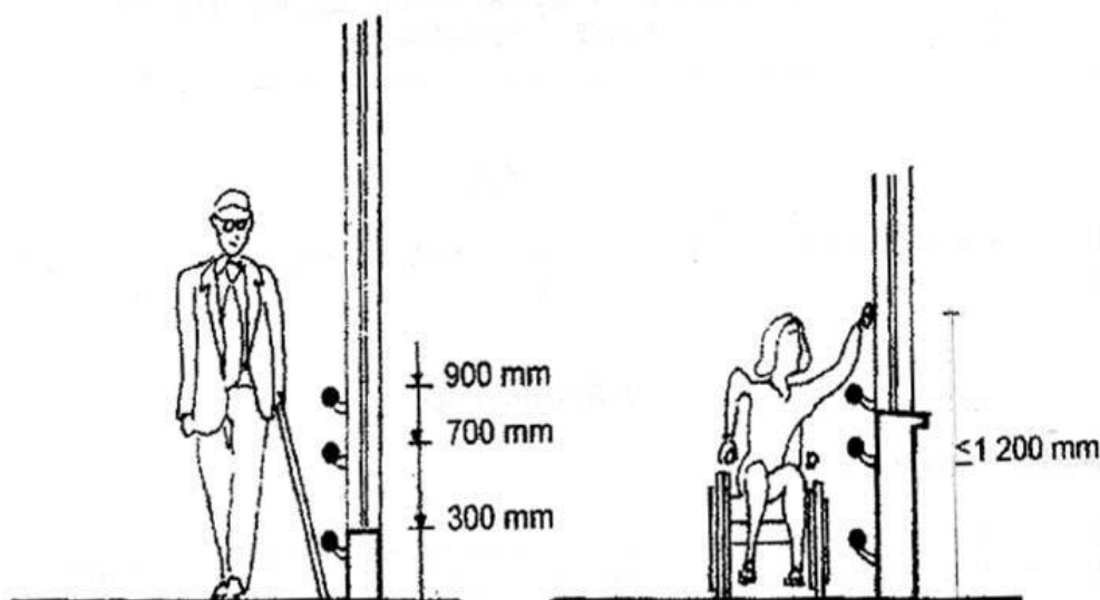
FIGURA 2. Pasamanos de protección en ventanas
